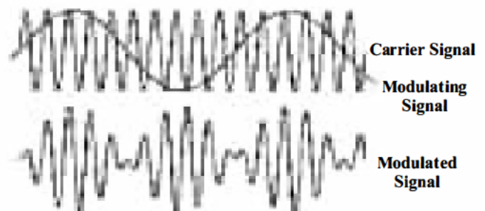
Fig: 14.9 Modulating
